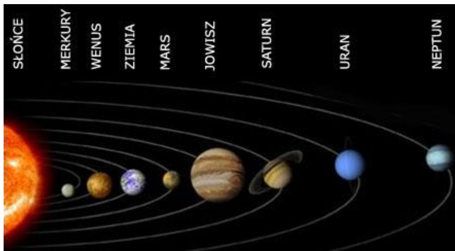
Układ słoneczny
